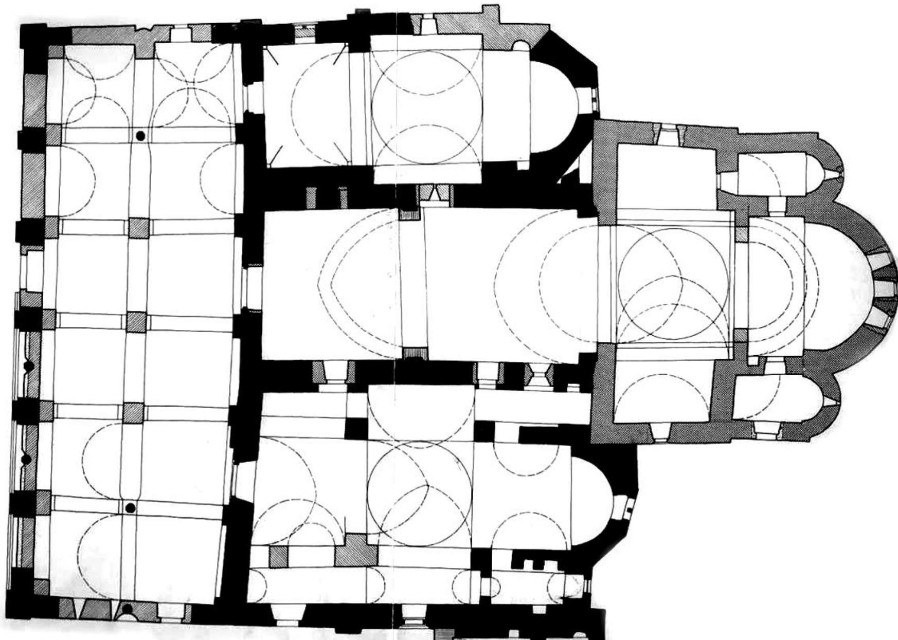
Peć, osnova, priprata na zapadu
