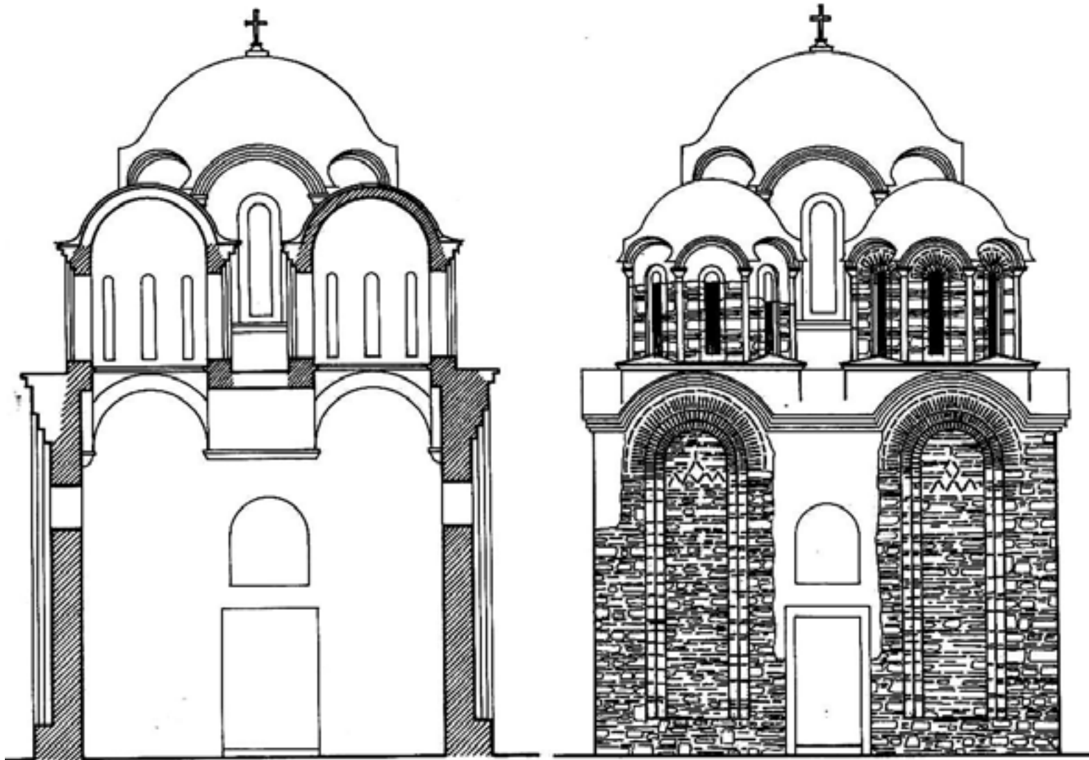
Velbužd, Sv. Spas, poprečni presek i rekonstrukcija zapadne fasade
