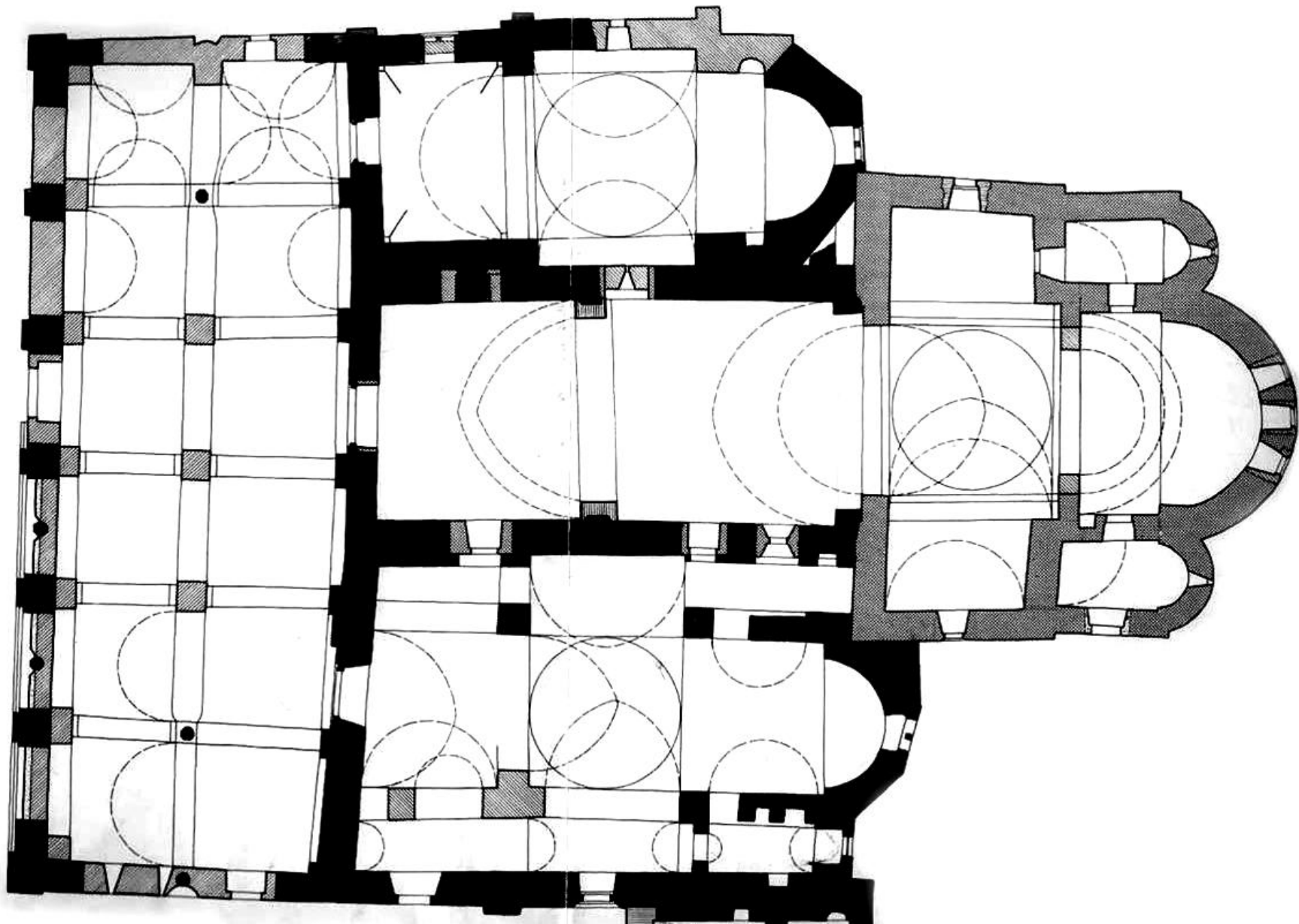
Peć, osnova, Sv. apostoli u sredini
