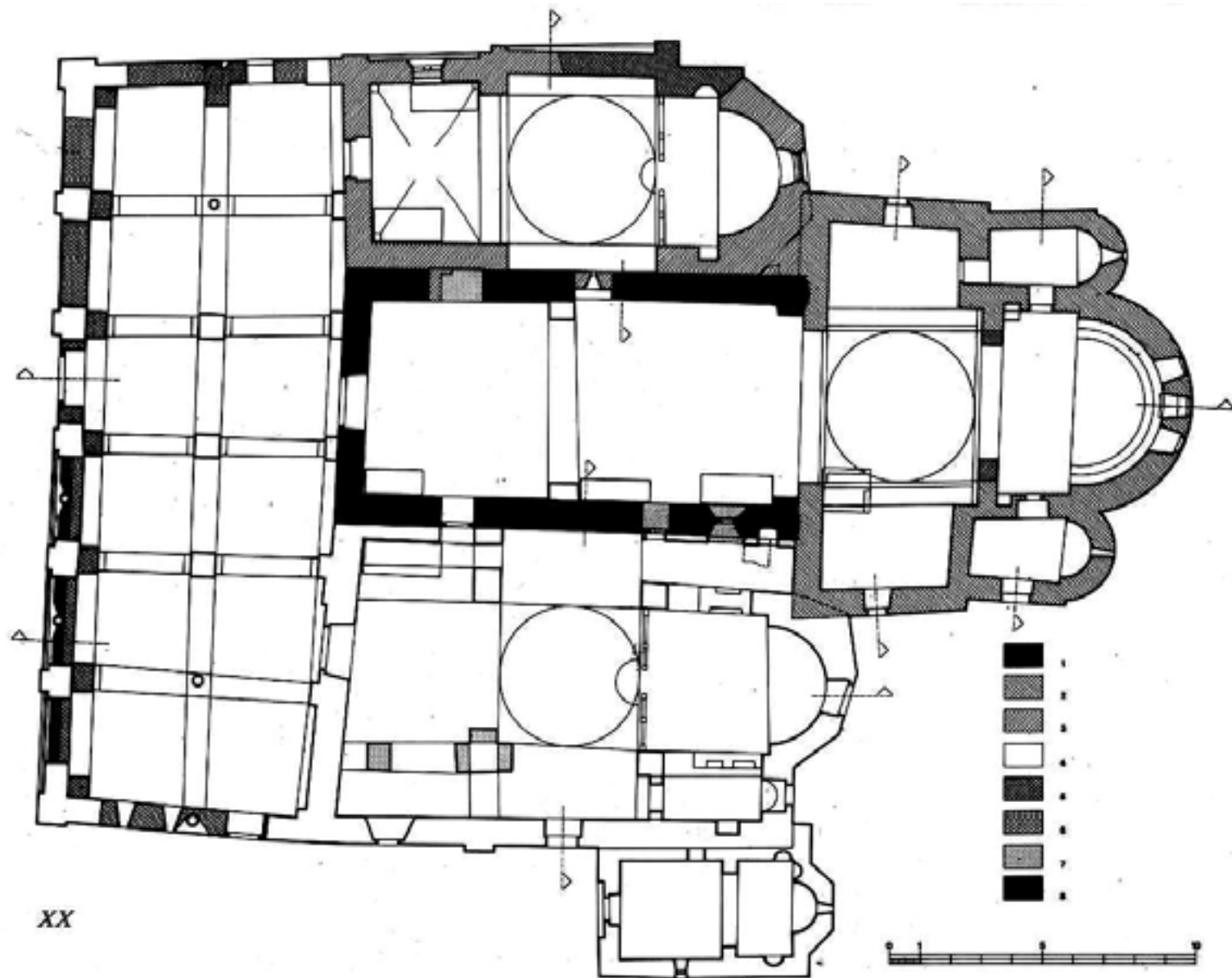
Peć, osnova, Sv. Dimitrije na severu
